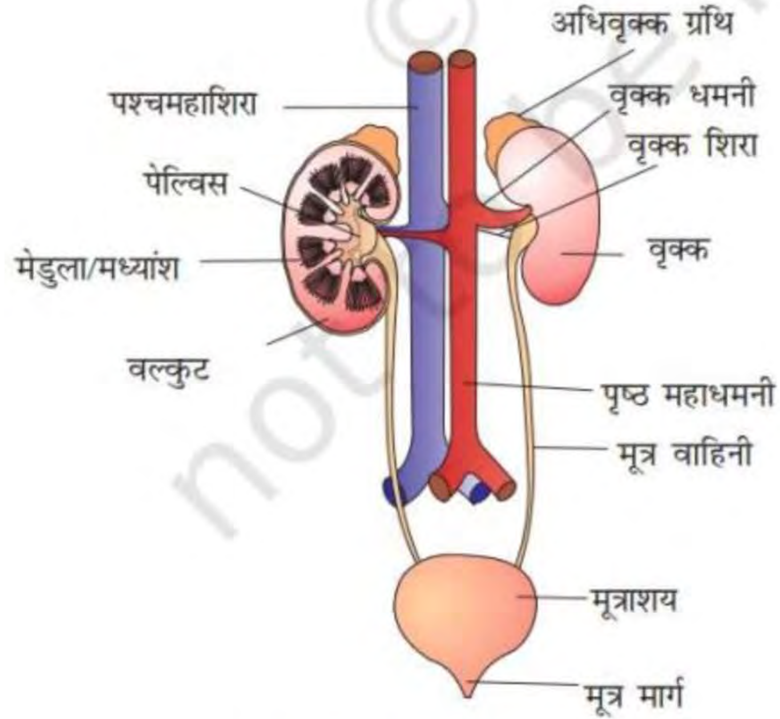
चित्र 19.1 मानव का उत्सर्जन तंत्र
